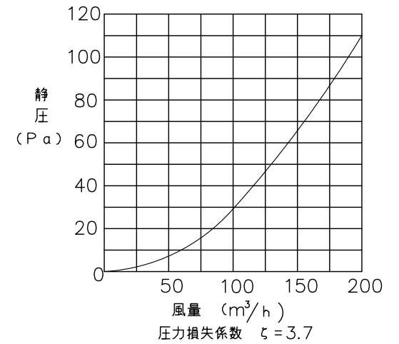
圧損特性
