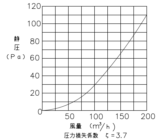
圧損特性
