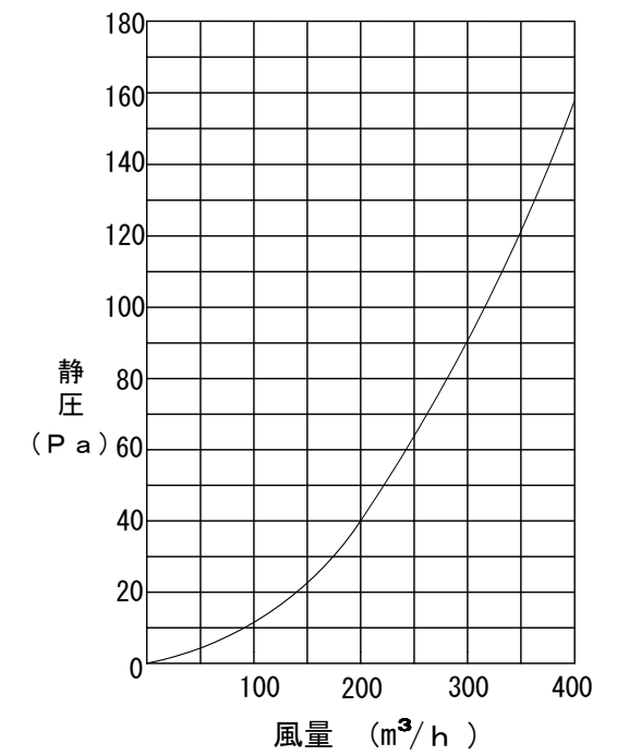
圧損特性
