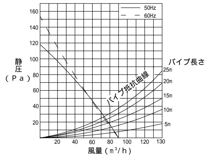
静圧曲線 抵抗曲線はVP管 100の場合
